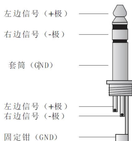
平衡或双声道1/4插头
