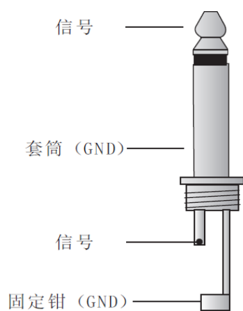
不平衡或单声道1/4插头
